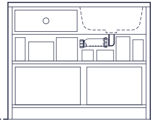
Dessous-lavabo avec une valve Hep v O installé horizontalement
