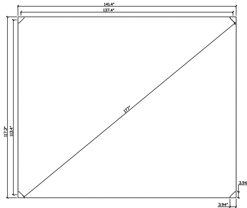
VUE DE LA BASE DE LA STRUCTURE VIEW OF STRUCTURE BASE
