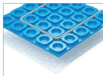
Sous-couche thermique de découplage de carrelage 1m x 1m / 1m x 5m / 1m x 15m
