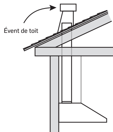
Évacuation verticale sur le toit
