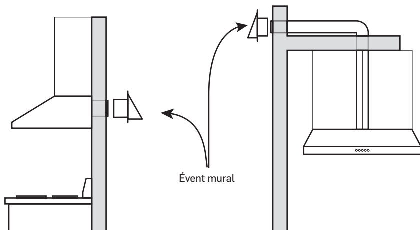
Évacuation horizontale au mur
