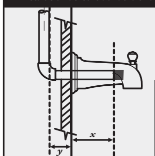
Instalación del surtidor de la tina
