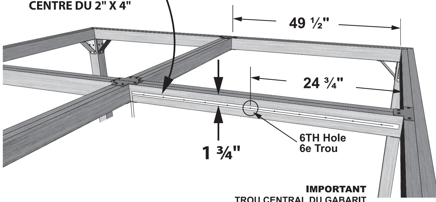
TEMPLATE / GABARIT
