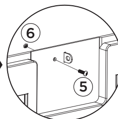
Vue extérieure Outside view
