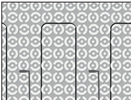
B. Localisation de la sonde dans le système de plancher chauffant avec membrane de désolidarisation. ( Installation 2 ème sonde optionnelle)
