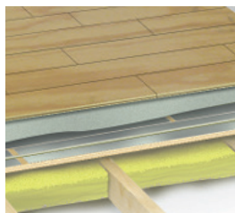
Sponplate 22mm med spor og varmfordelingsplater
