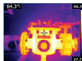
Uten isoleringskappe
