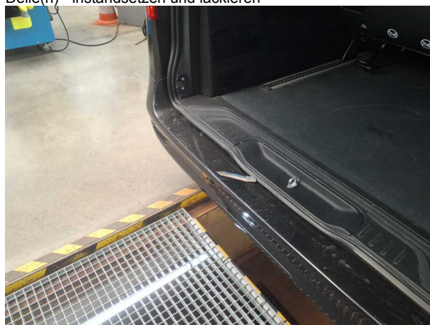
Beschädigung #7: Stossfänger hinten: Stossfänger mit Parktroni... verformt - erneuern
