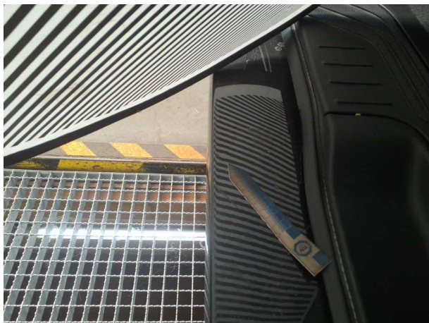
Beschädigung #7: Stossfänger hinten: Stossfänger mit Parktronic - verformt - erneuern
