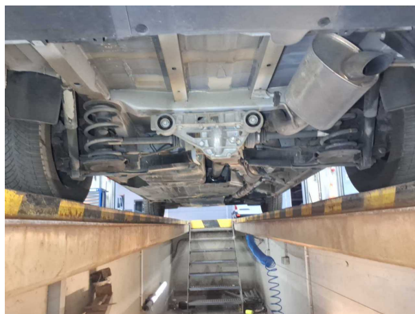
Abbildung 8: Unterboden
