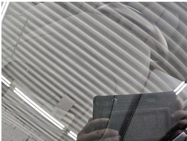
Frontscheibe Steinschlag mit Riss (DEKRA)
