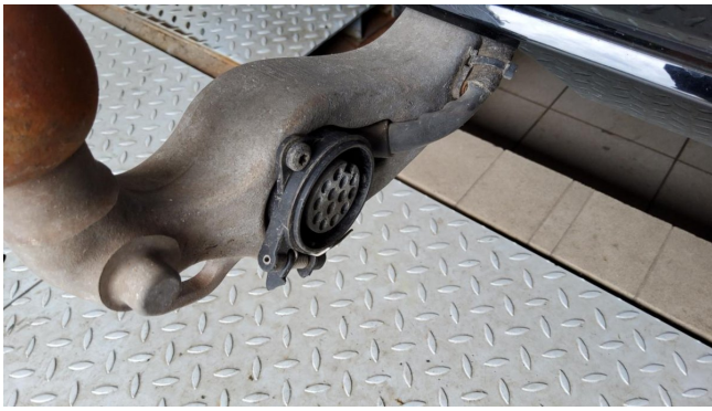
AHK Steckdose beschädigt ern.
