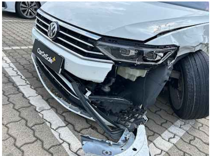
Stoßstange vorne (Riss/Bruch, Verformung)
