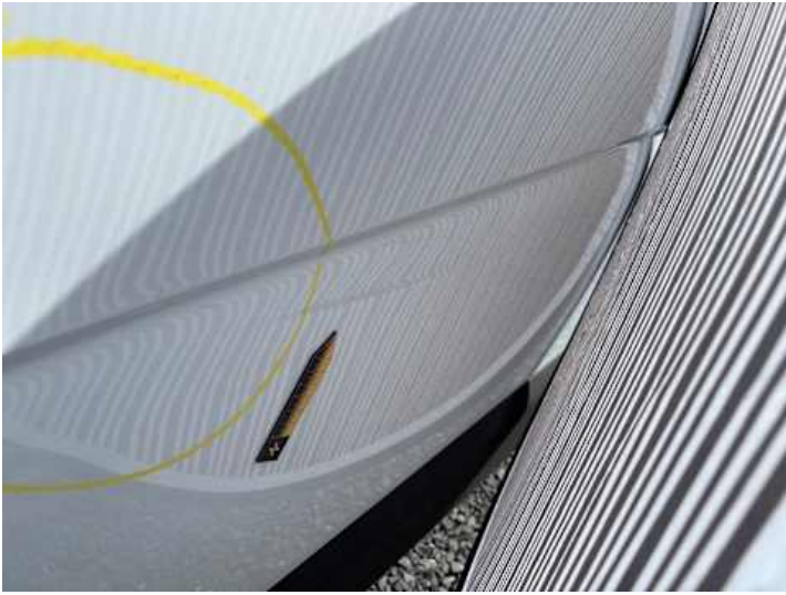
Türe hinten rechts (Spaltmaße ungenau, Verformung)
