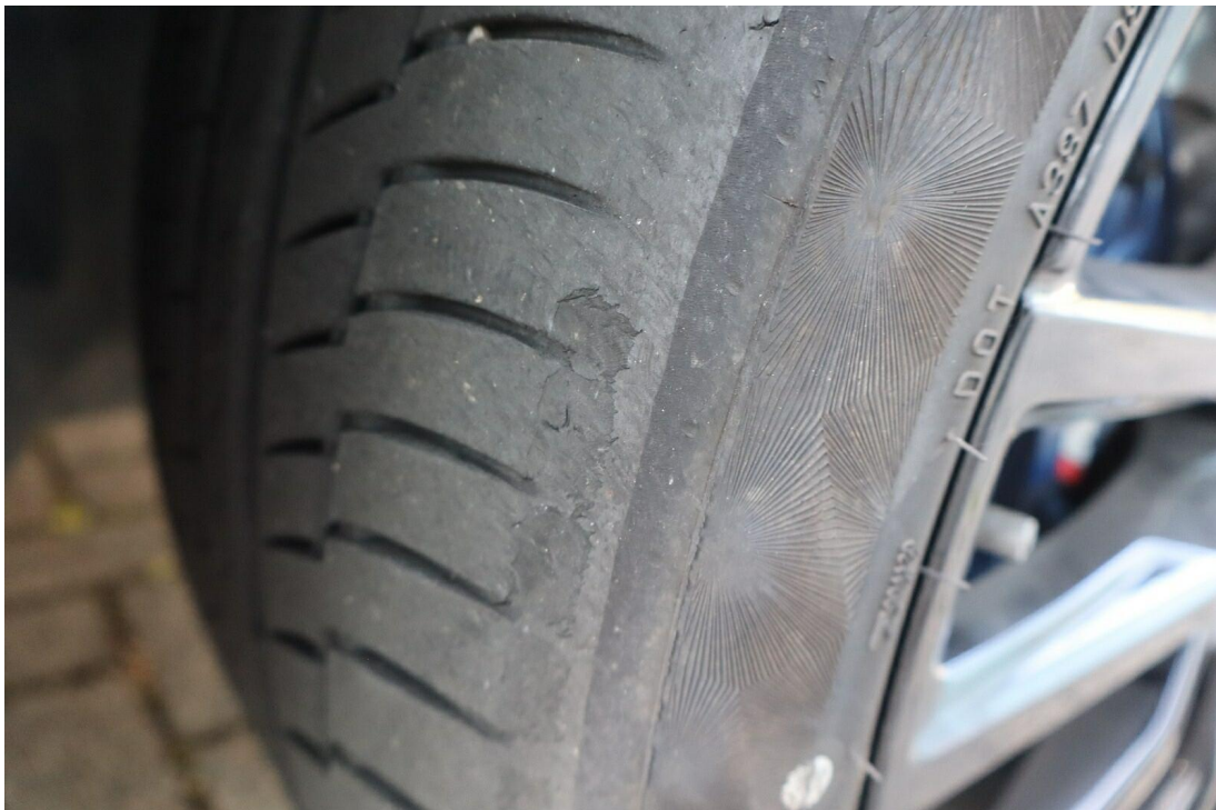
Bild 12 : Reifen vorn stark einseitig abgefahren
