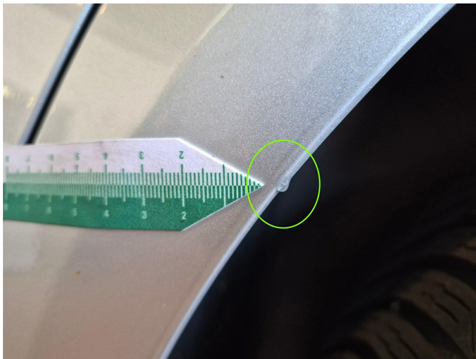
Bild 11 : Seitenwand hinten links erhebliche Applikationsfehler im Radlaufbereich (Tropfenbildung)
