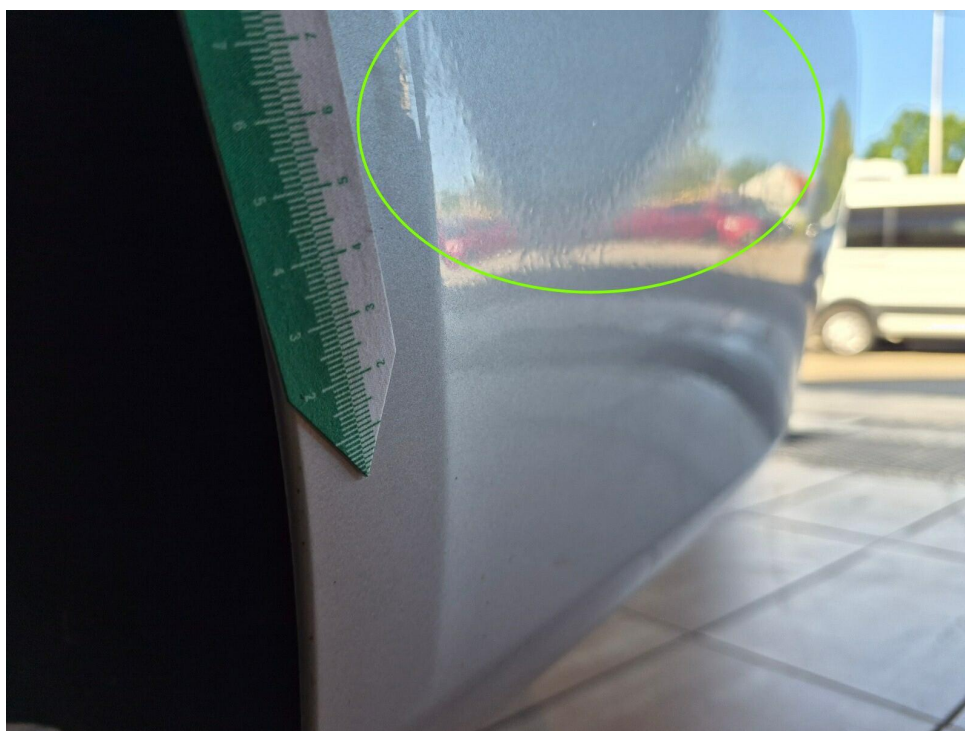
Bild 12 : Stoßfängerverkleidung hinten erhebliche Applikationsfehler (Orangenhaut)
