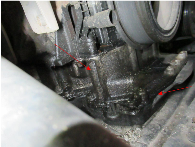
Bild 9: Technik, Motor - Undichtigkeit, Freitext, prüfen und Befund festlegen, Schadenerweiterung möglich
