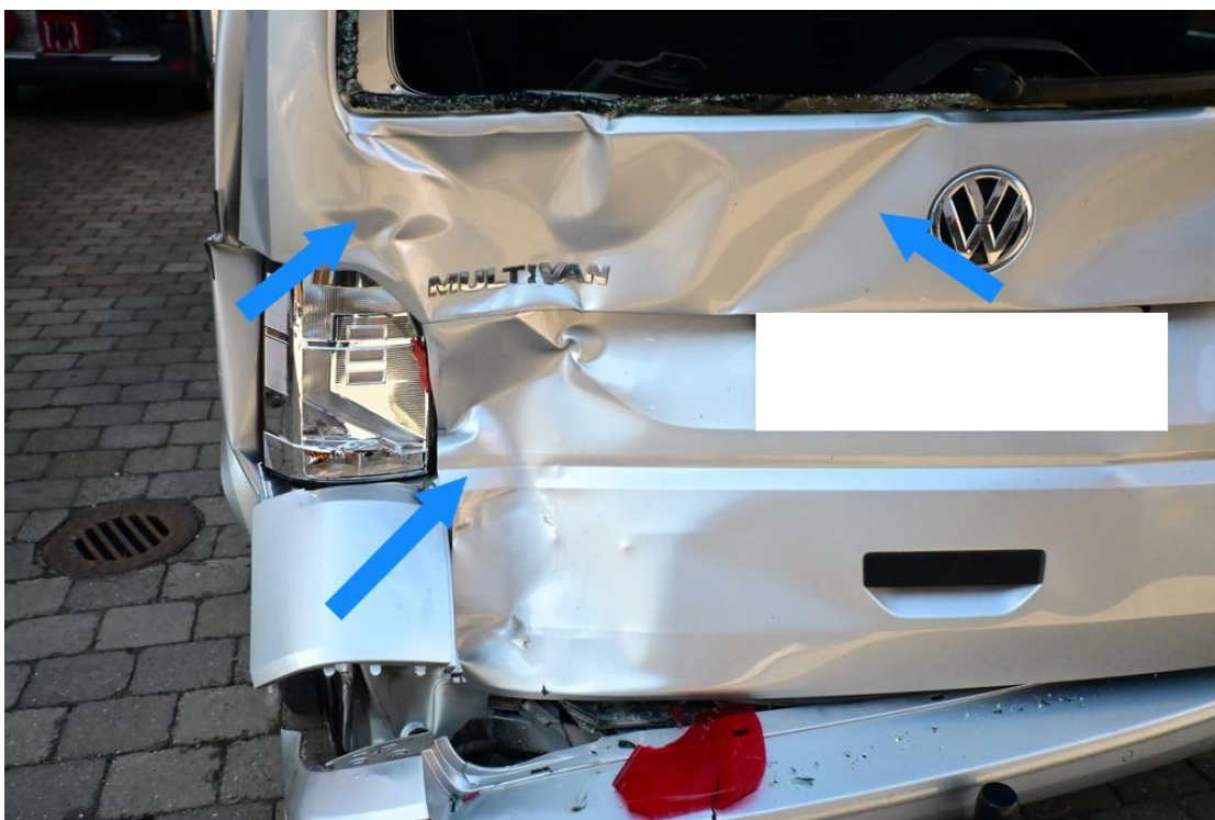
Bild 12 - Heckklappe deformiert
