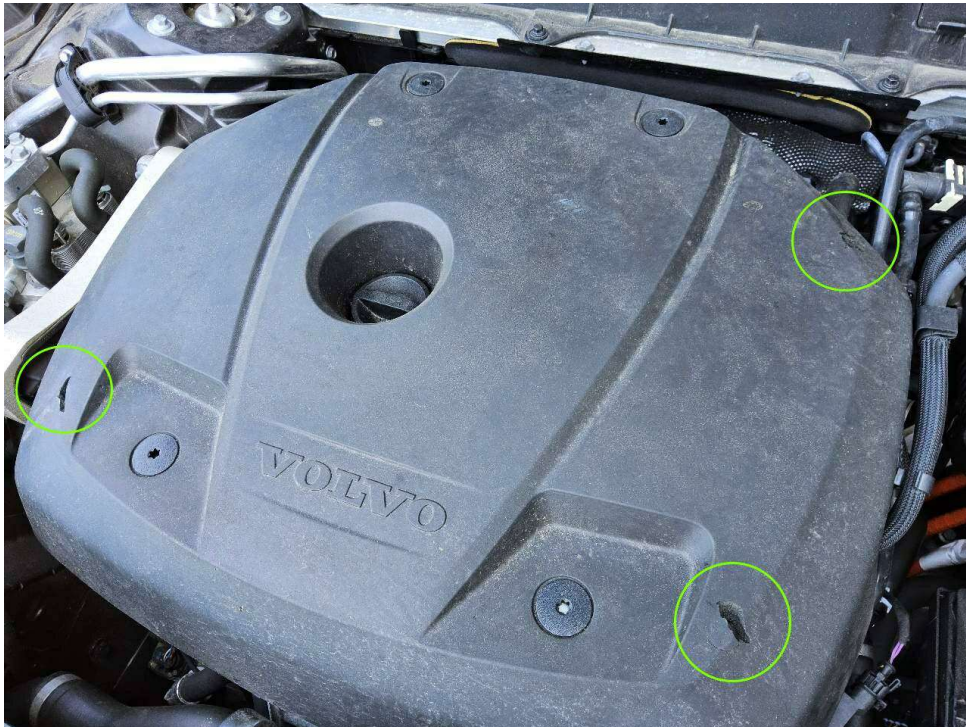
Bild 9 : Motorabdeckung Tierversbiss
