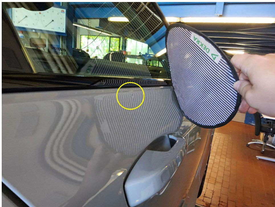
Bild 18 : Tür vorne rechts oberhalb eingedellt
