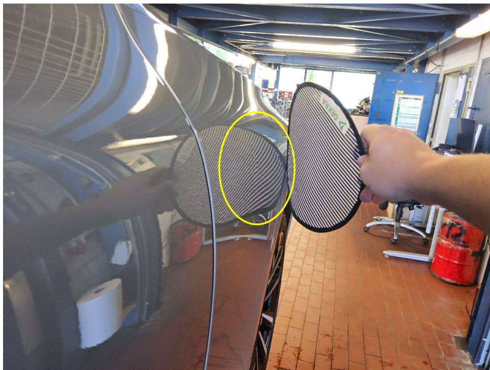
Bild 19 : Kotflügel vorne rechts eingedellt und verschrammt
