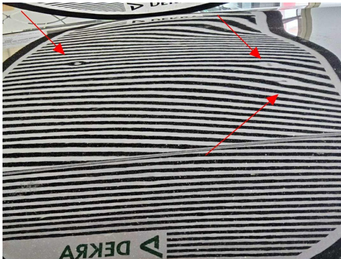
Bild 17: Außen, Dach, mehrfach eingedellt, drücken
