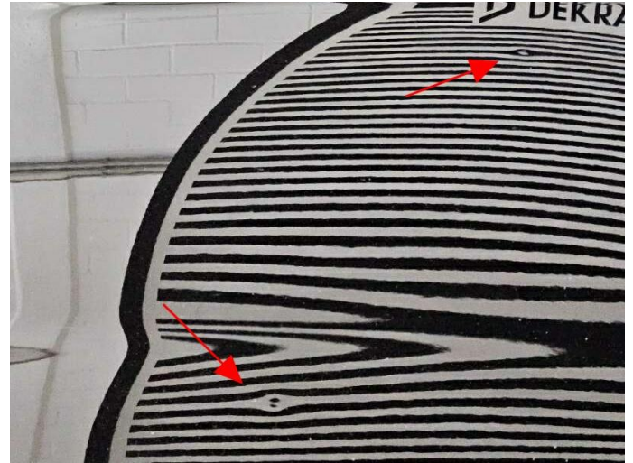
Bild 22: Außen, Motorhaube, mehrfach eingedellt, drücken
