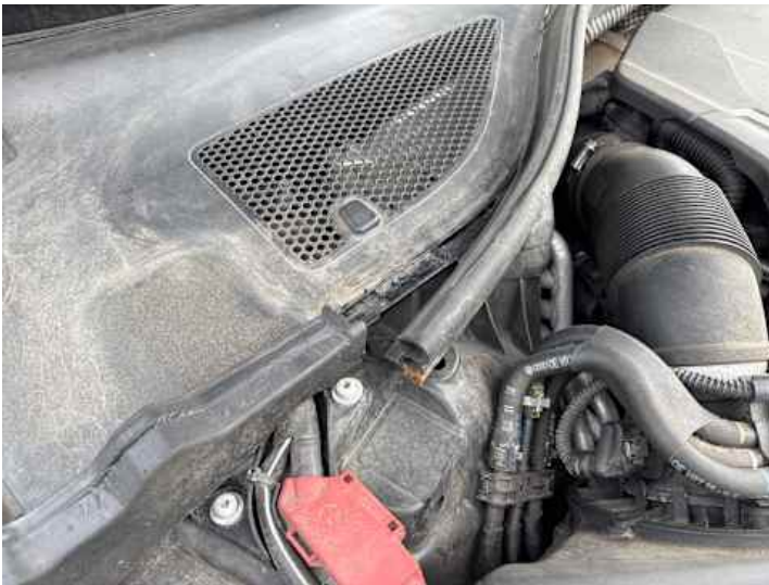
Motorhaube (Riss/Bruch)
