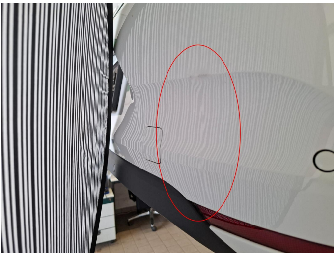
Bild 7: Außen, Stoßfänger hinten, verformt, erneuern
