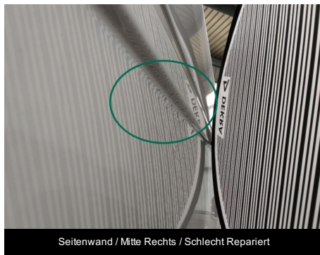
Seitenwand / Mitte Rechts / Schlecht Repariert
