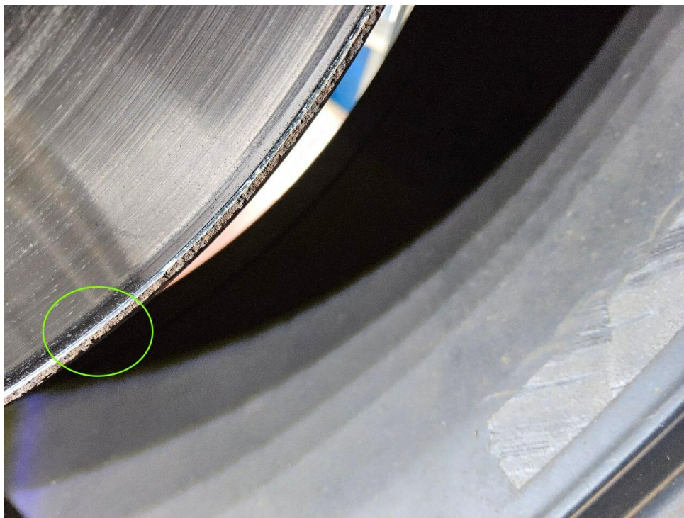
Bild 40 : Bremsscheiben und Bremsbeläge Hinterachse verschlissen
