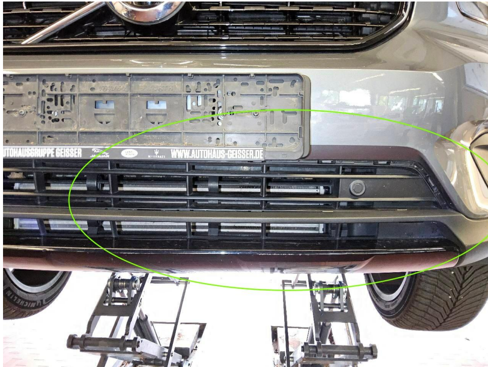
Bild 25 : Anfahrtschaden vorne links, Kühlergrill unten eingedrückt und Diffusor glanzschwarz verschrammt
