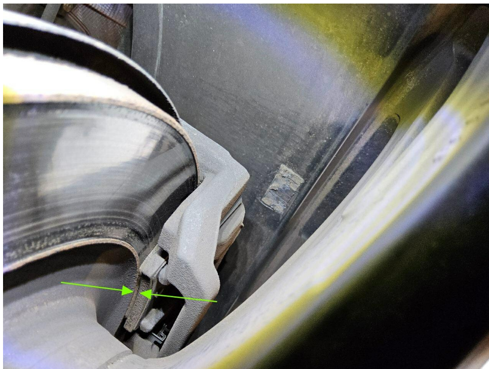
Bild 39 : Bremsscheiben und Bremsbeläge Hinterachse verschlissen
