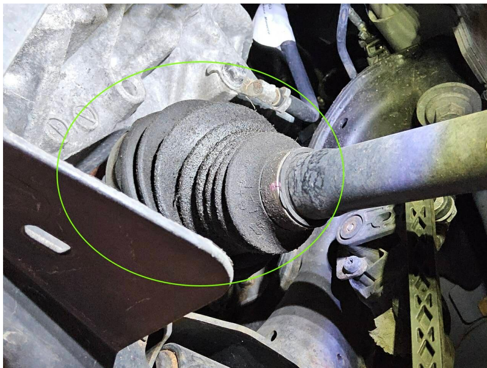
Bild 41 : Antriebswellen Vorderachse, Manschetten innen ölfeucht / fettig
