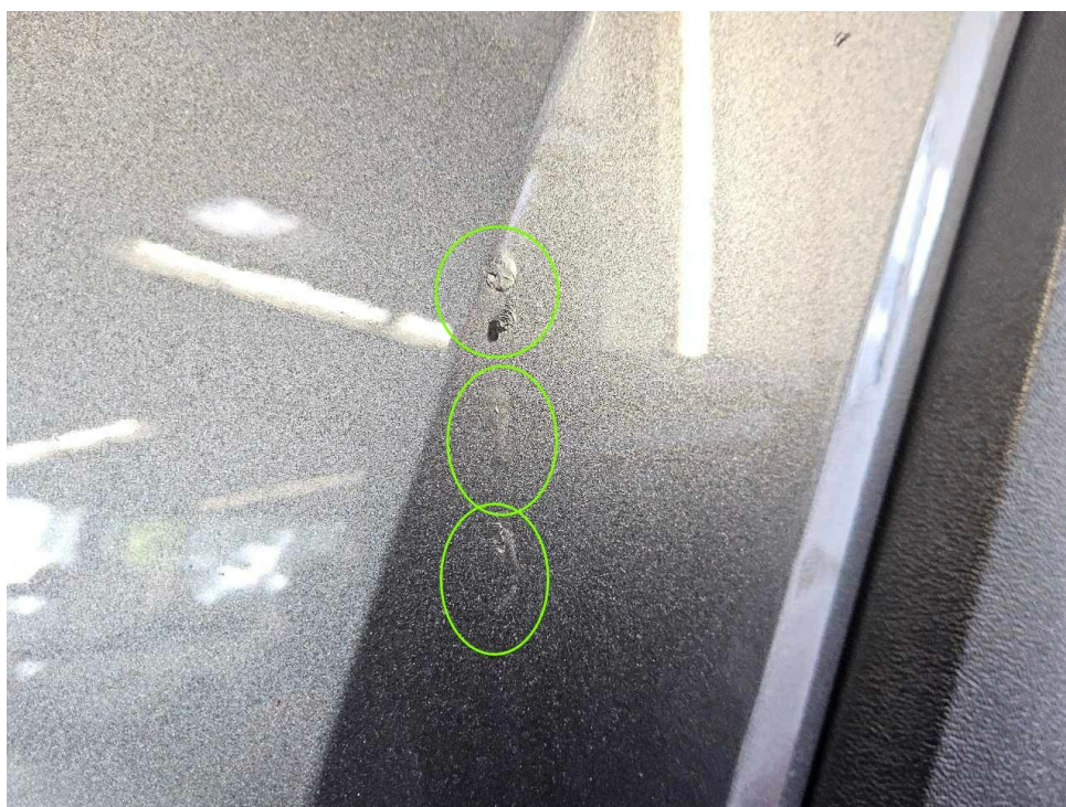
Bild 24 : Stoßfänger vorne leichte Steinschläge und leichte Kratzer, leichte Lackanätzung und links verschrammt
