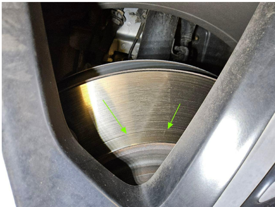
Bild 37 : Bremsscheiben Vorderachse verschlissen
