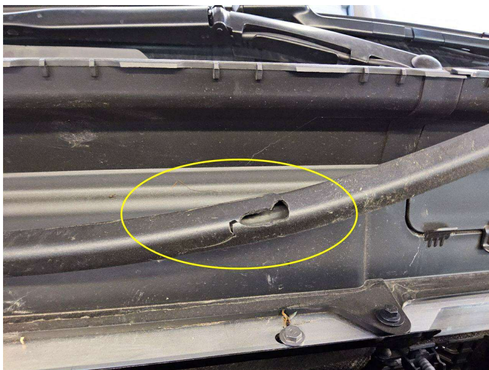
Bild 12 : Motorraumabdichtung links, mittig und rechts Tierversbiss
