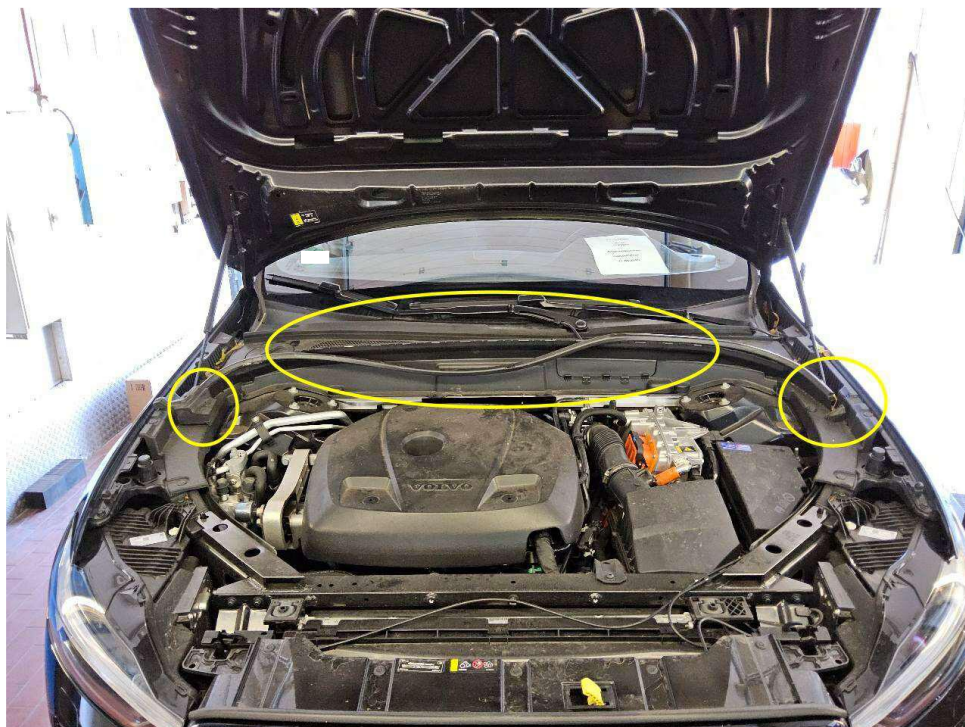
Bild 10 : Motorraumabdichtung links, mittig und rechts Tierverbiss
