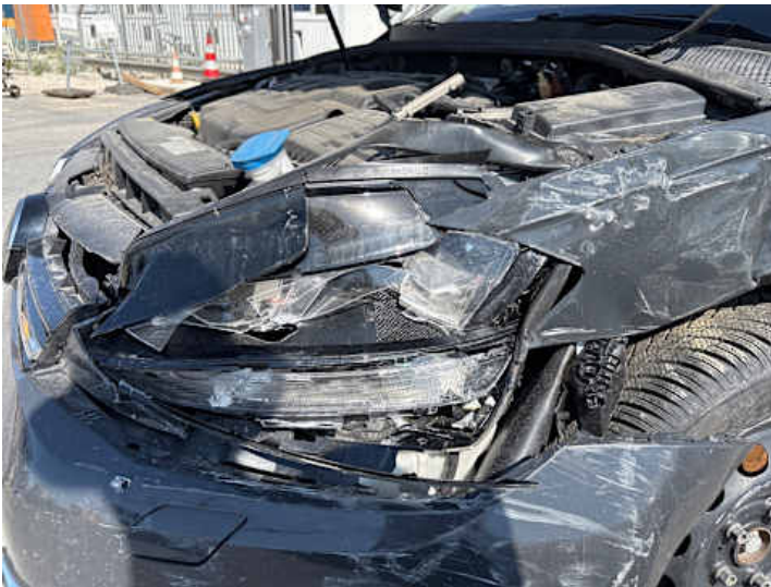
Scheinwerfer (links) (Riss/Bruch, Ohne Funktion)
