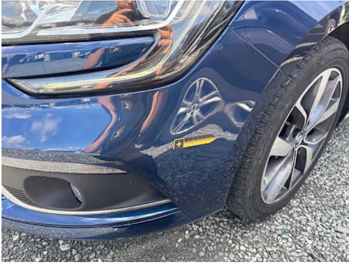
Stoßstange vorne (Verformung)
