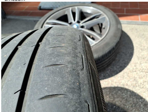
Beschädigung #8: 2.Radsatz: 2 Reifen (Außenprofil) - verschliss... - erneuern
