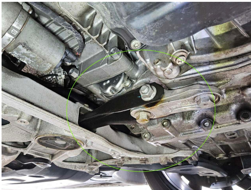
Bild 30 : Motor / Getriebe ölfeucht überprüfen und lokalisieren
