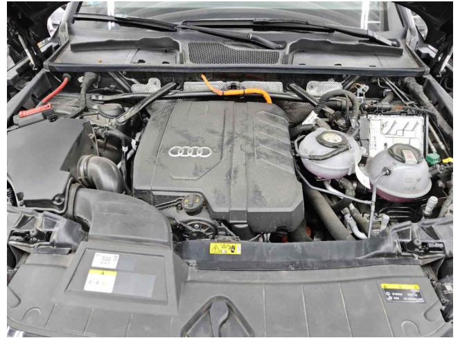
Motorraum (DEKRA)
