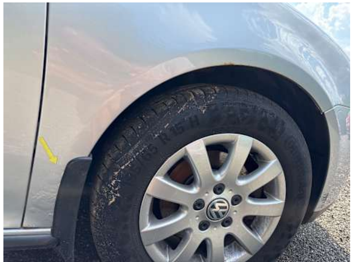
Kotflügel vorne rechts (Rost)
