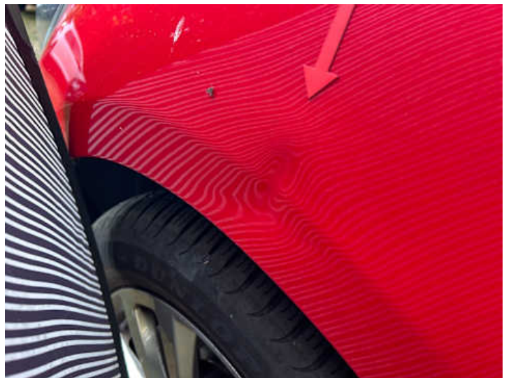
Fahrtür (Verformung)
