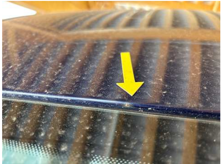
Dach (Rost)
