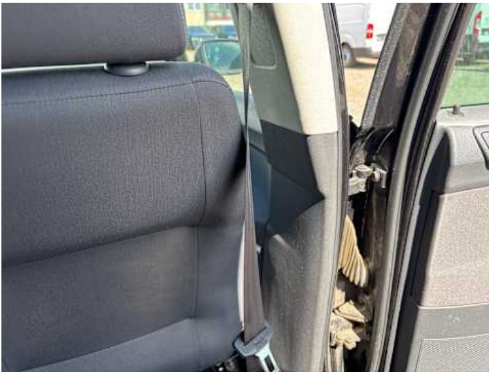
Innenraum (Anderer Schaden): Gurtstrafer defekt
