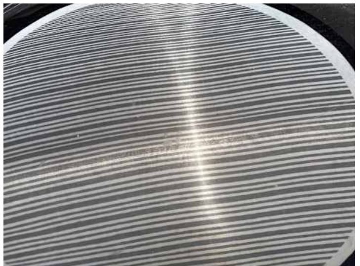
Motorhaube (Lackschaden)
