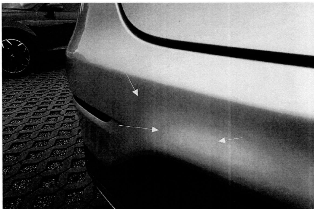
Bild 6 : Stoßfänger verschrammt und plastisch verformt
