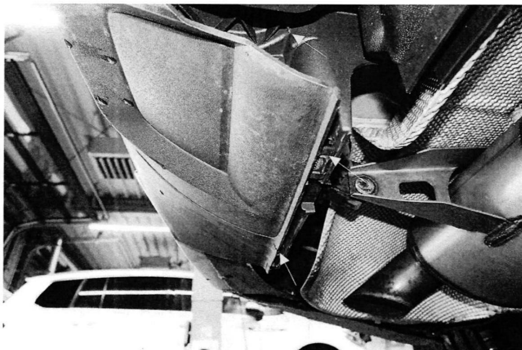
Bild 11 : Aufnahme Unterteil unten ausgebrochen
