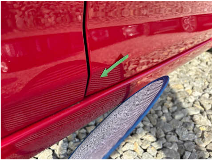
Beifahrertür (Verformung)
