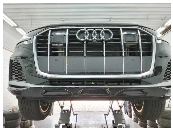
Frontspoiler, Luftführungsgitter mit Blende und Schließteil beschädigt (gebrochen) (DEKRA)
