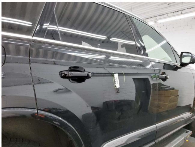
Tür hinten rechts unsachgemäß lackiert, Orangenhaut und Silikoneinschlüsse (DEKRA)
