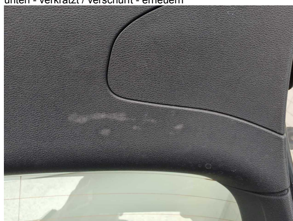
Beschädigung 5: Heckklappe/-tür: Verkleidung Standard unten - verkratzt / verschürft - erneuern
