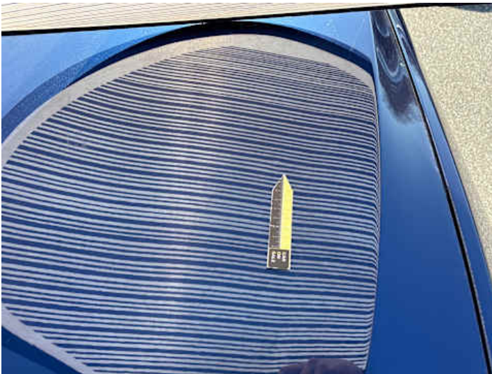
Motorhaube (Delle)
