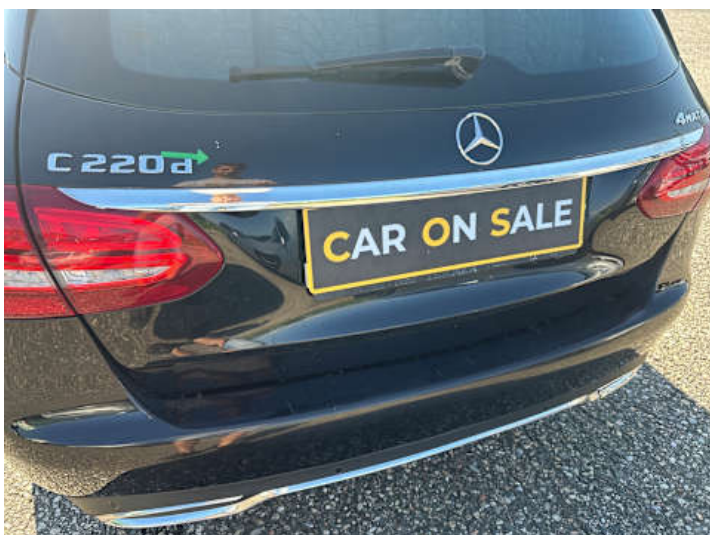
Heckklappe (Lackschaden)
