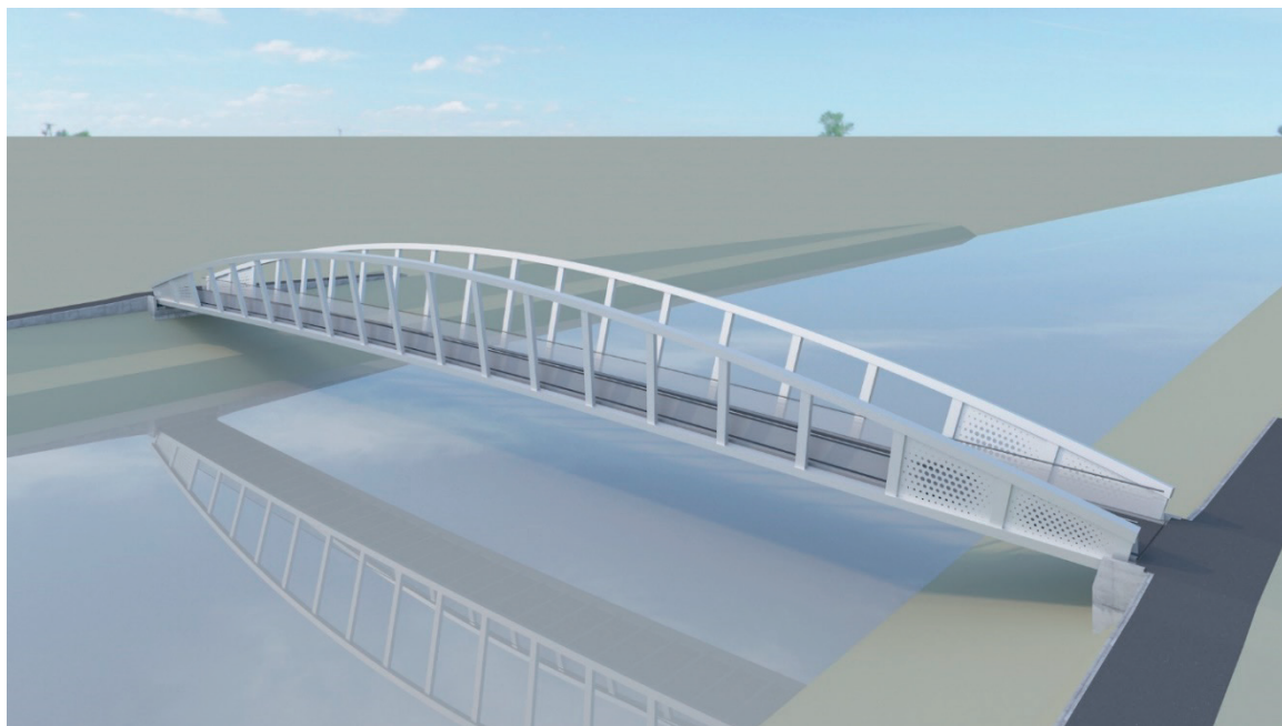
Grafika brvi čez Savinjo pri Špici v okviru kolesarske povezave Celje - Žalec (Vir: povzeto iz spletne strani MOC)
