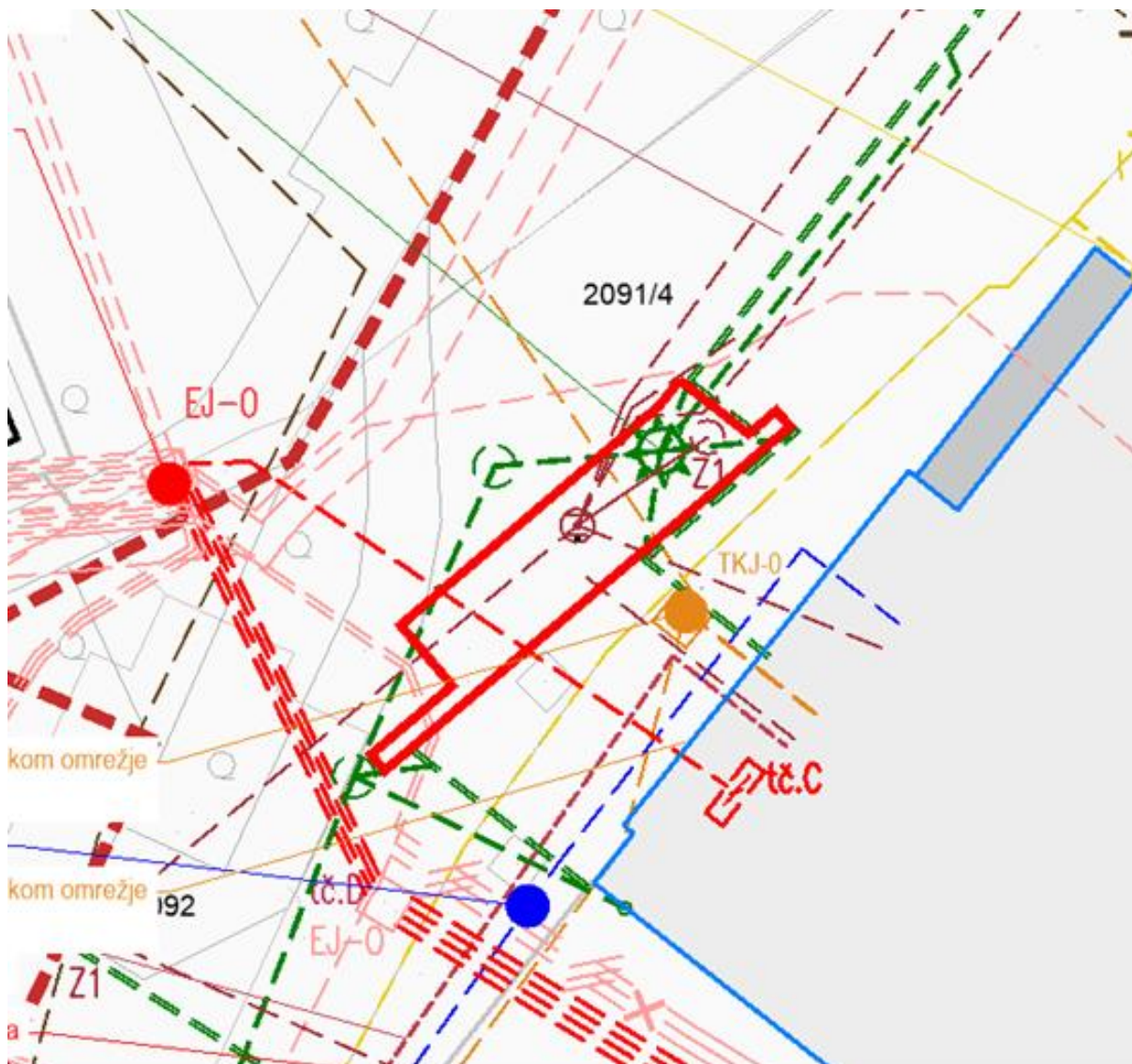
Slika 9a: Izrez iz situacije komunalnih vodov: kanalizacija, vključno s ponikovalnico (zelena), javna razsvetljava (temno rdeča) in elektrika (svetlo rdeča). Vir: projektant kombinat.arhitekti, Ljubljana
