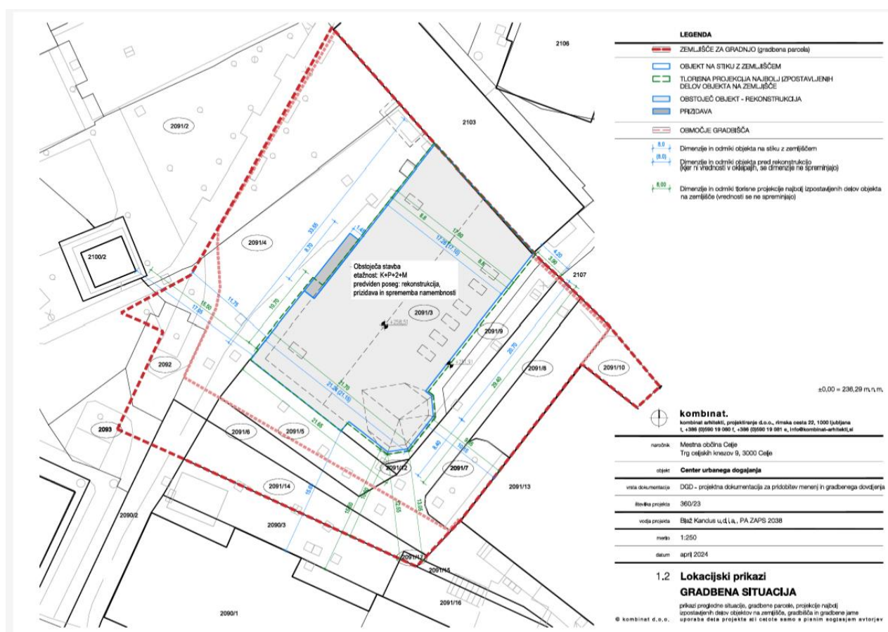
Slika 9: Izrez iz gradbene situacije/okolice , Vir: projektant kombinat.arhitekti, Ljubljana
