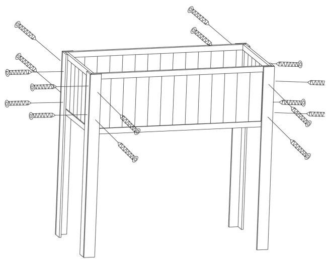
Schrauben 3,5 x 30 mm (16 Stück) Screws 3.5 x 30 mm (16 pieces)
