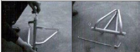
Togliere la vite dal supporto e rimuovere il mandrino.
