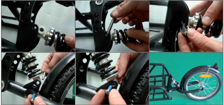
Montare l'ammortizzatore al telaio di sostegno.
