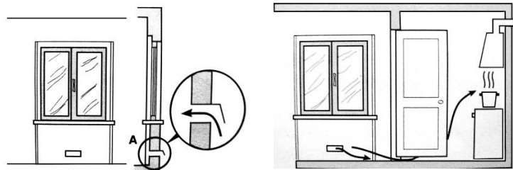
Beispiel für Zulufteöffnungen für die Verbrennungsluft
