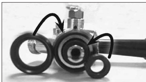
Joints sur la partie inférieure du coupleur de CO 2
